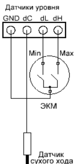
Рис.11 ЭКМ любых исполнений
