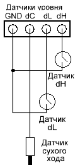
Рис.13 Поплавковые датчики любых типов (датчик dC – электродный)
