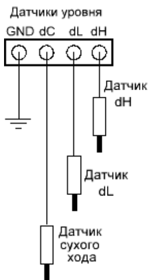
Рис.12 Электродные датчики
