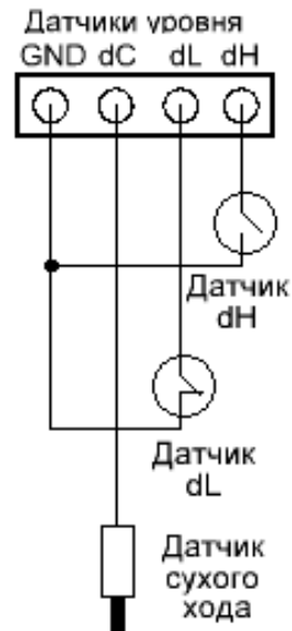
Рис.13 Поплавковые датчики любых типов (датчик dC – электродный)
